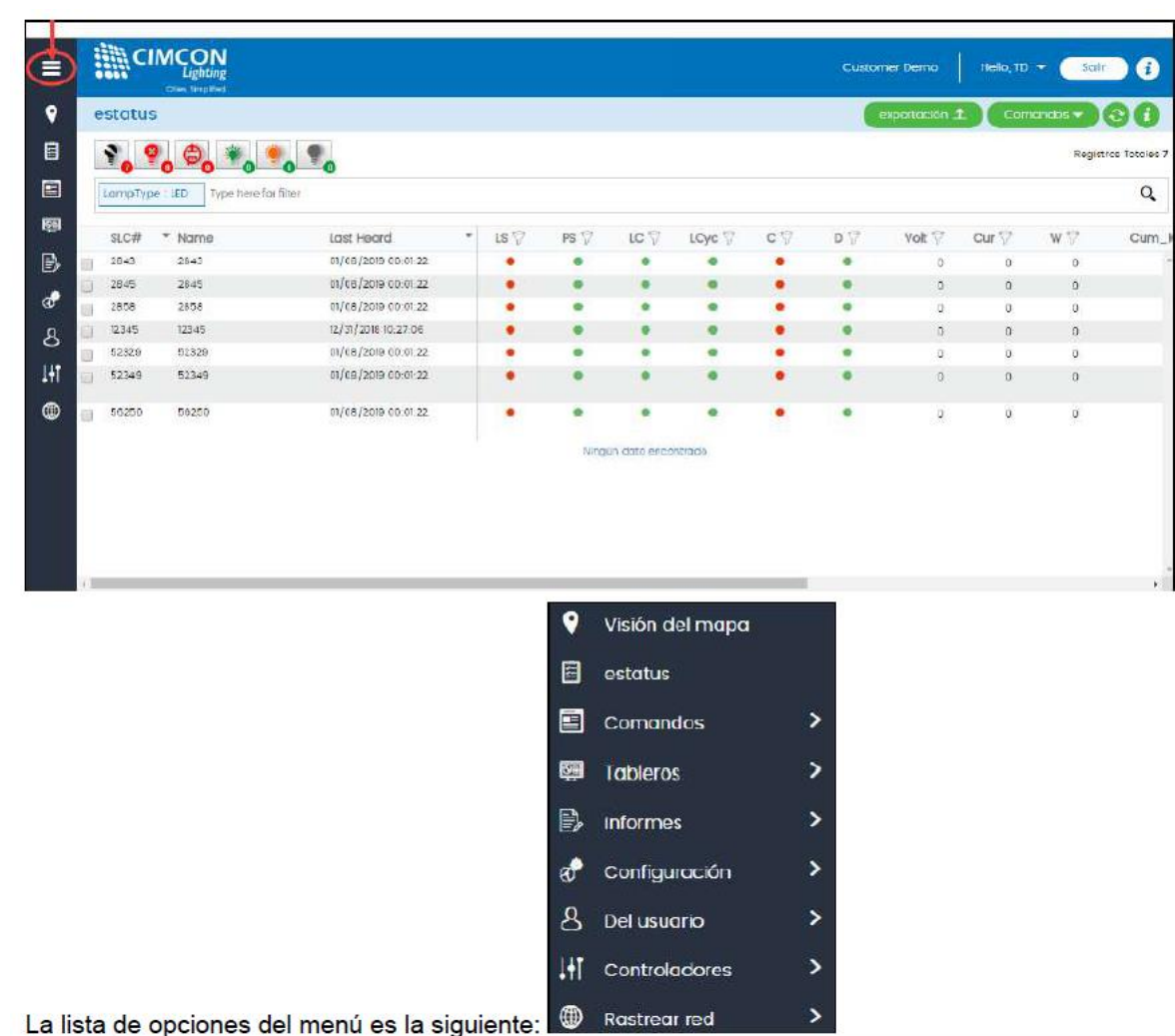
Gráfica 45. Sistema LG V5 Quantela
