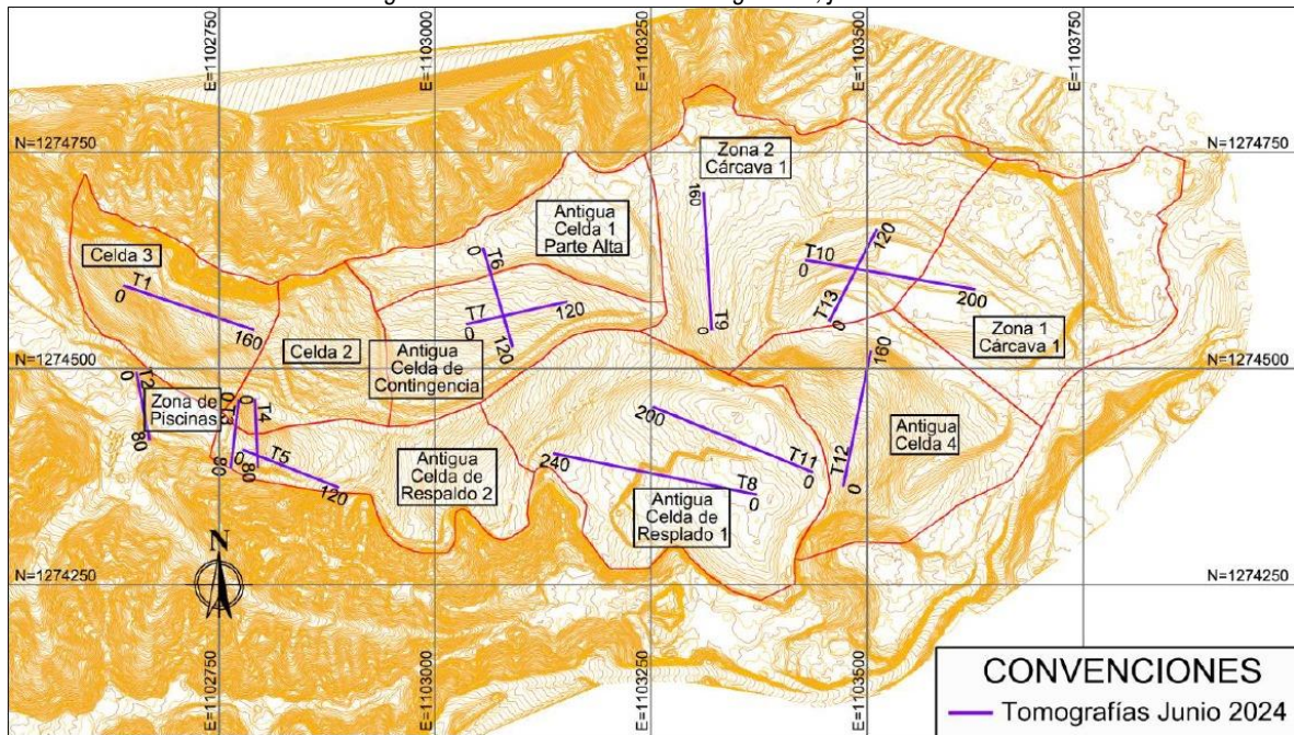
Figura. Localizaciones líneas tomograficas, junio 2024
