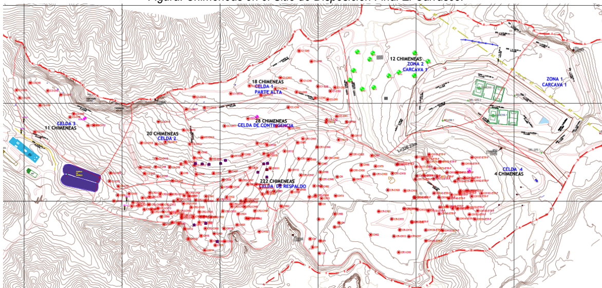
Figura. Chimeneas en el Sitio de Disposición Final El Carrasco.
