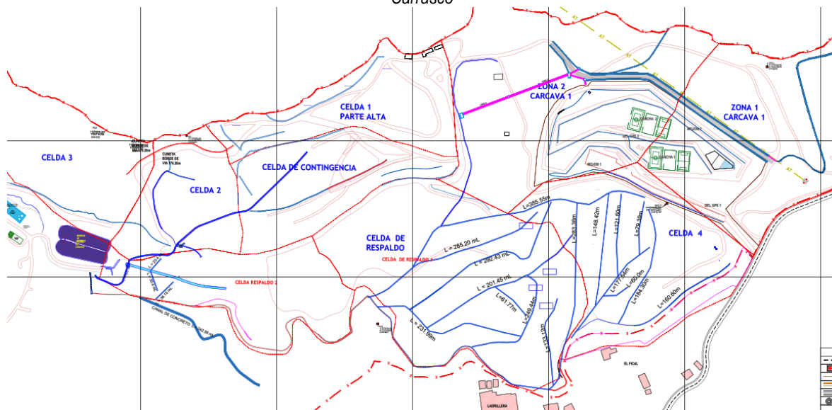
Figura. Panorámica del estado actual de los canales para la conducción de las aguas de escorrentía en El SDF "El Carrasco"
