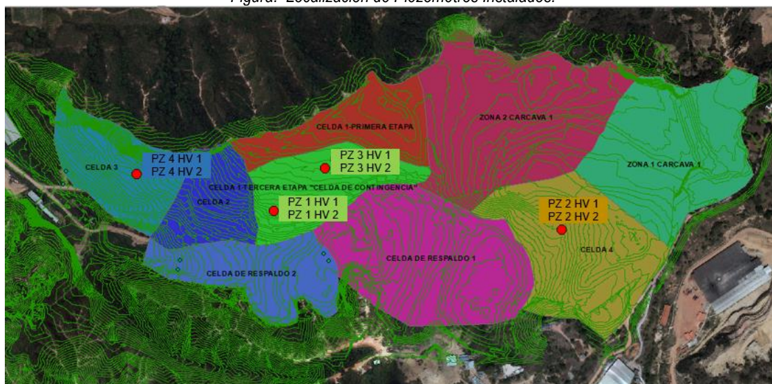
Figura. Localización de Piezómetros Instalados.
