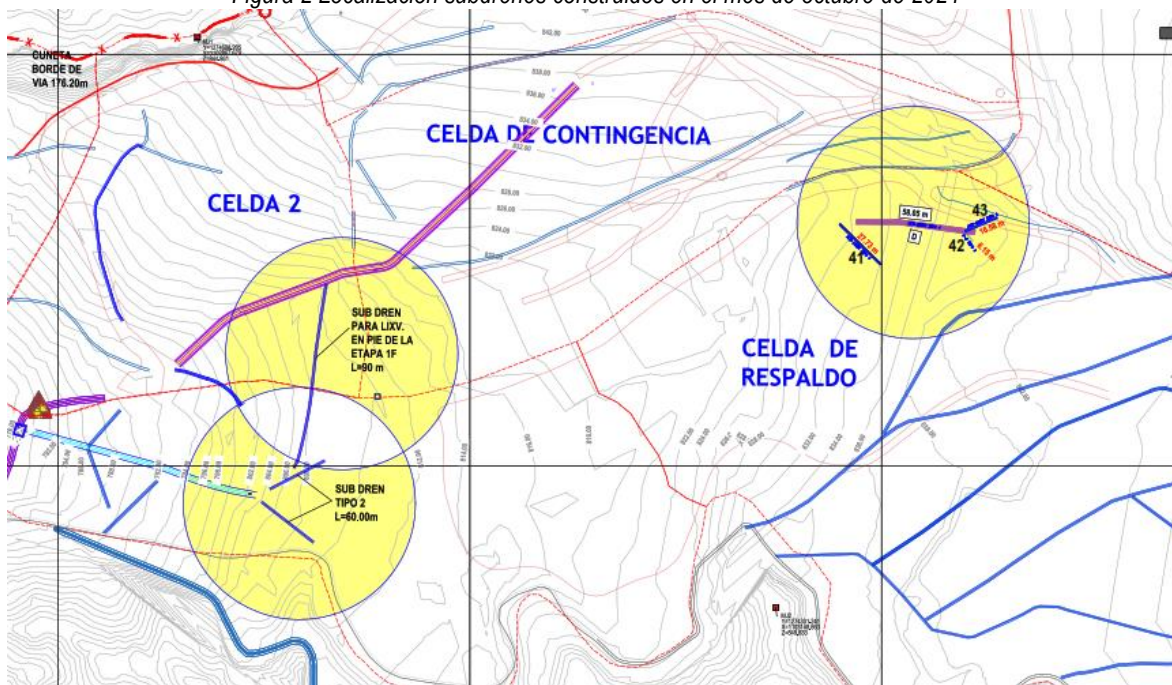
Figura 2 Localización subdrenes construidos en el mes de octubre de 2024
