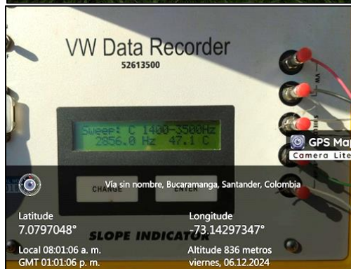
Ilustración. Lectura de Piezómetros de hilo vibrátil
